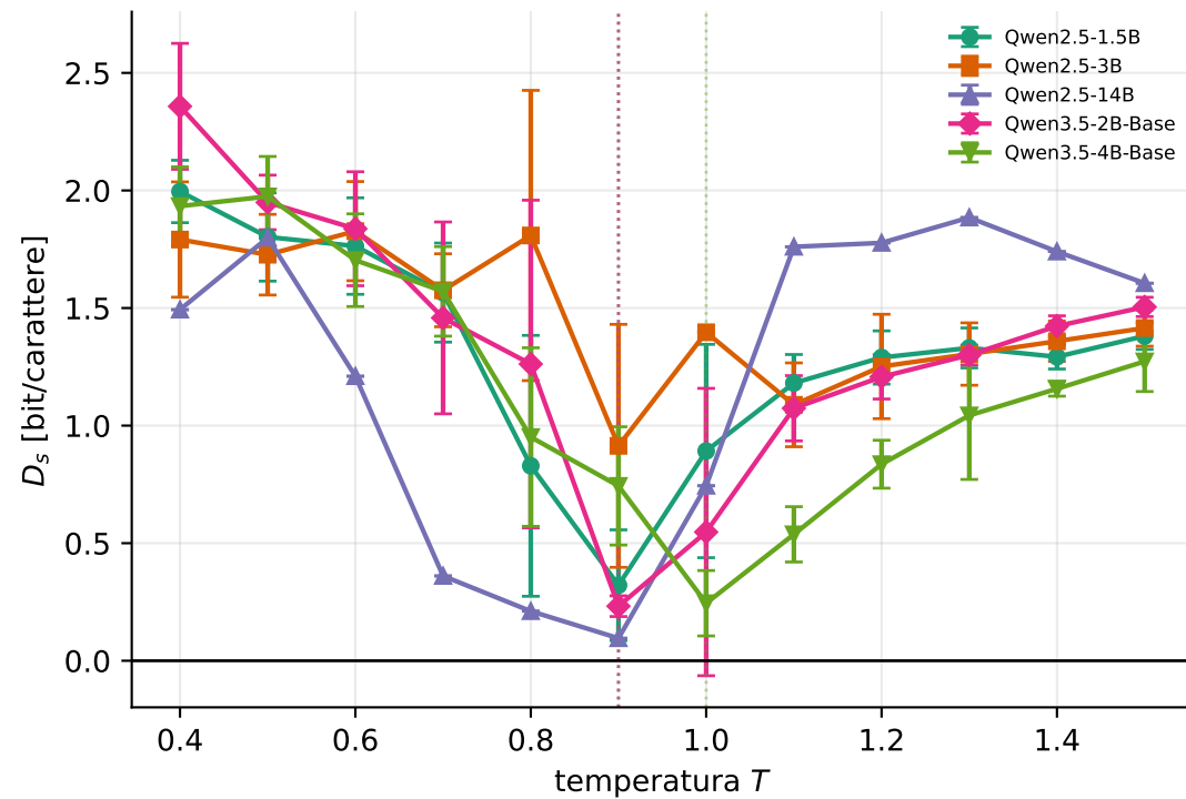
Divergenza KL simmetrizzata dal testo umano il minimo dà T^* (cfr. [L] Fig. 5A)
