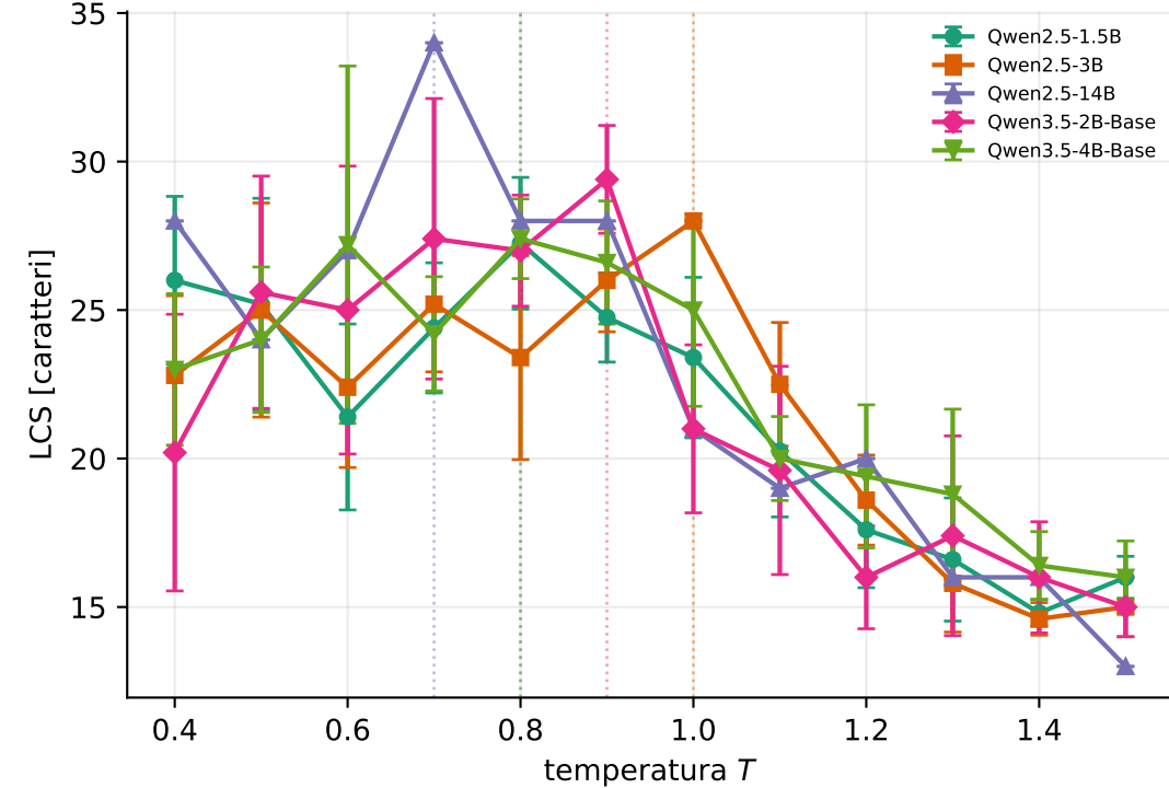
Sottostringa più lunga in comune con Tolstoj (cfr. [L] §III-D)
