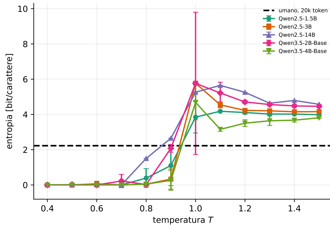
Entropia stimata per compressione (cfr. [L] Fig. 5B)
